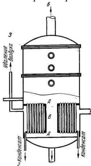
2- сурет Тігінен орналасқан құбырлы вакуумды аппарат
