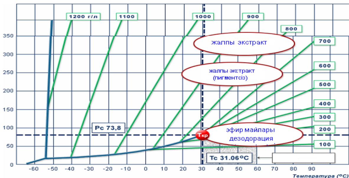
2-сурет Жоғары критикалық флюидті экстракция параметрлері
