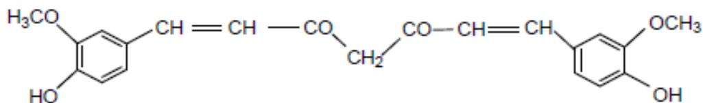
Куркумин
