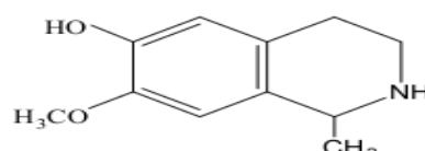
Сальсолин
