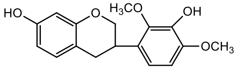
мукронулактон
