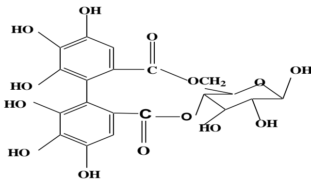
4,6-(-)-гексагидроксидифеноил-β-Д-глюкоза
