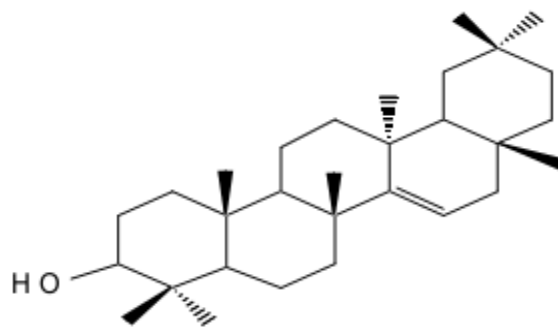
Тараксерол (1.25)
