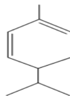
Фелландрен
