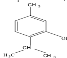
Тимол
