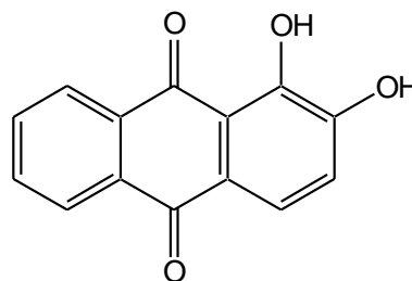
Ализарин
