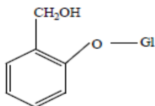
Салицин
