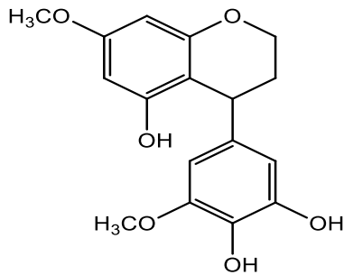
5,3',4'-триокси-7,5'-поинсеттиолан
