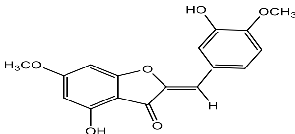
4,3'-диокси-6,4'-ауреусидин I
