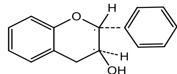
(-) - катехин
