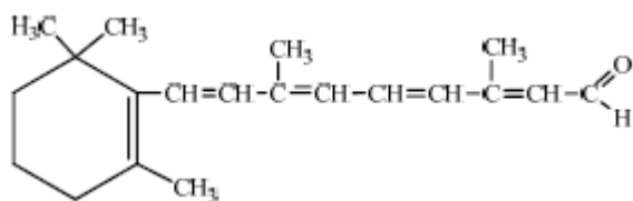
Тұтас транс-ретиналь
