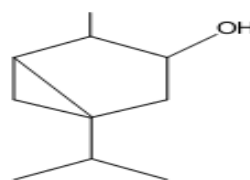
Туйол
