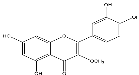
5,7,3',4'-тетрагидрокси-3-метоксифлавоноид (5-зат)
