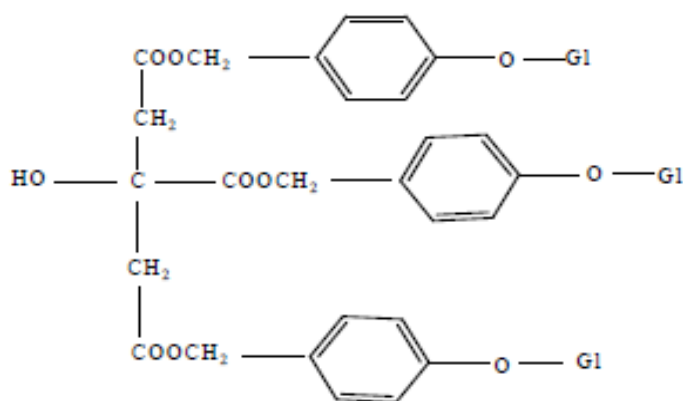
Паришин
