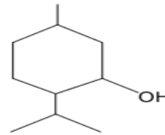
Ментол
