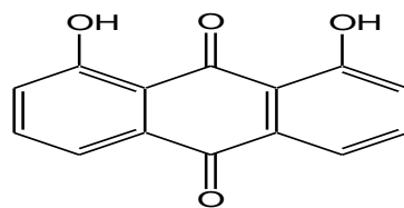
Хризацин
