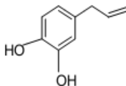
Аллилпирокатехин
