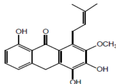
Целебиксантонқышқылы
