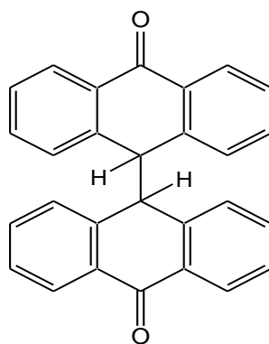
диантрон
