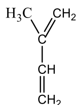
Изопрен
