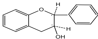
(-) - эпикатехин
