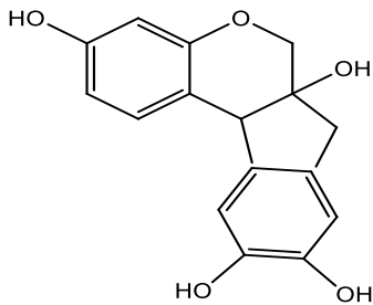
бразилин
