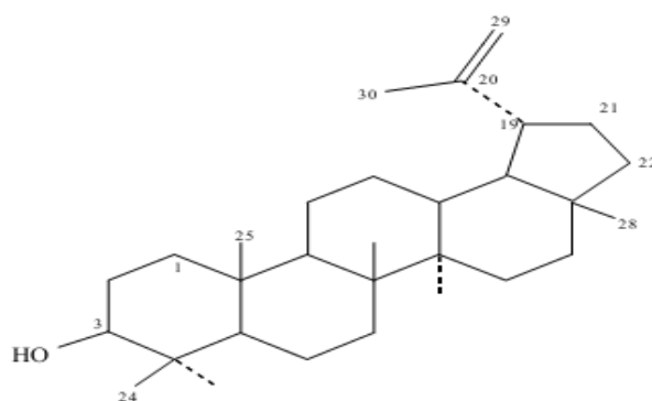
Лупеол (Лупан)
