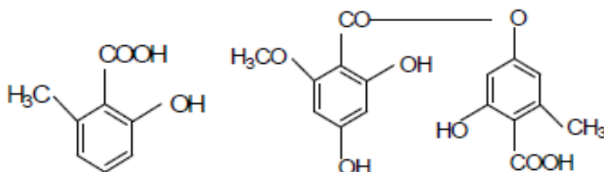
Орселлин қышқылы
