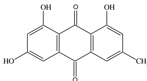
ЭМОДИН
