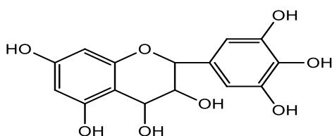
лейкодельфинидин
