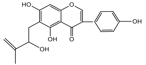
лабкретин
