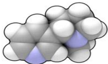
Никотин C_{10}H_{14}N_2
