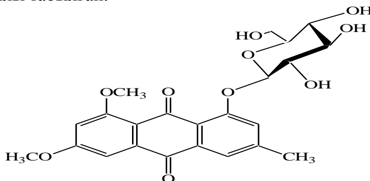
6,8-диметокси-3-метилантрахинонның 1-О-β-D-глюкопиранозиді
