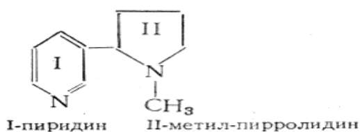
Никотин
