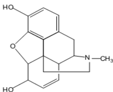
Морфин
