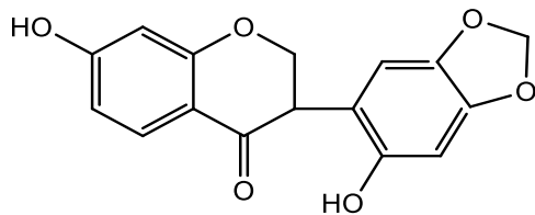
софорол
