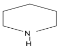
Пиперидин
