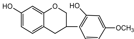
веститон
