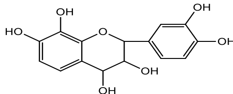
мелакацидин
