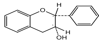
(+) - эпикатехин
