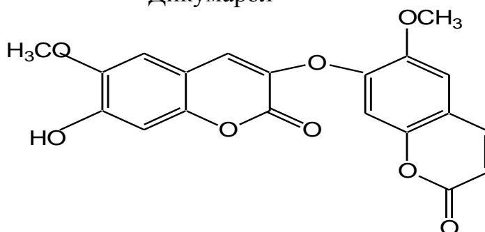
Дикумарол
