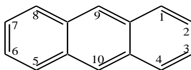
антрацен
