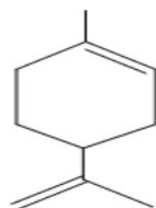
Лимонен
